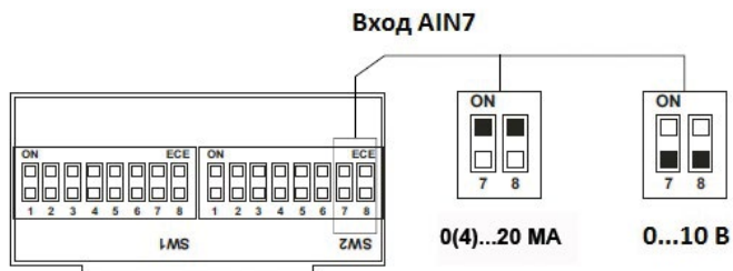
Рисунок Б1.22 - выбор типа входного сигнала DIP переключателями
