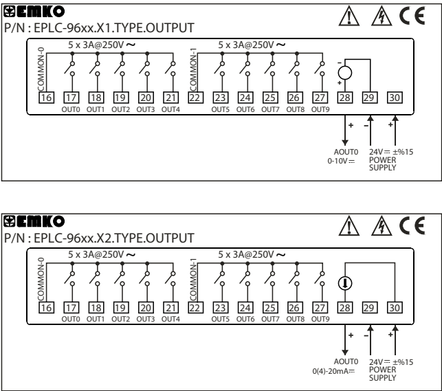
Рисунок Б2.14 - Общая схема подключения модуля вывода «тип X»
