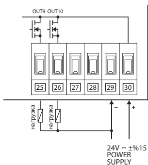
Рисунок Б2.9 - схема подключения нагрузки
