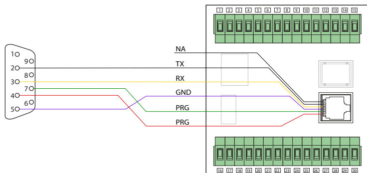
Рисунок 15.1 - Схема распыки кабеля программирования
