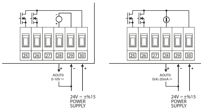
Рисунок Б2.7 - схема подключения аналоговых выходов
