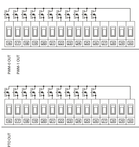
Рисунок Б2.6 - схема расположения PWM/ПТО выходов
