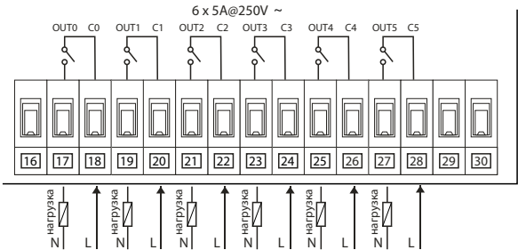
Рисунок Б2.18 - схема подключения нагрузки к релейным выходам
