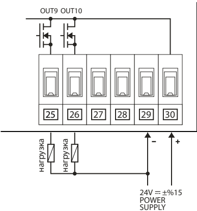
Рисунок Б2.5 - схема подключения нагрузки
