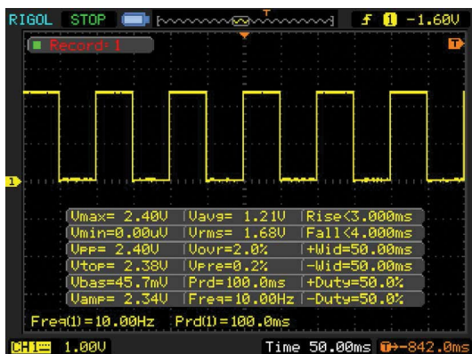
Рисунок В.2.1 — PTO режим работы
