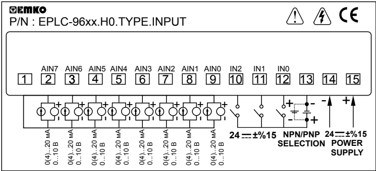
Рисунок Б1.18 — общая схема модуля «тип Н»
