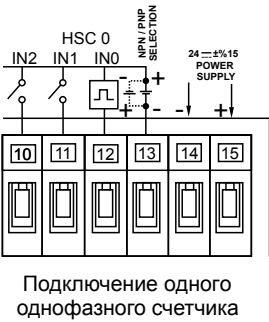
Рисунок Б1.17 — схема подключения одного высокоскоростного счетчика (HSC)
