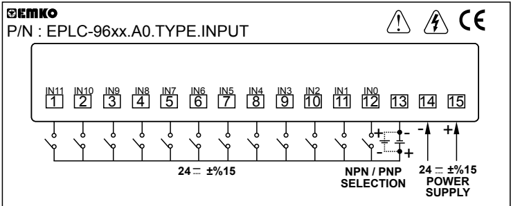
Рисунок Б1.1 - общая схема модуля «тип А»
