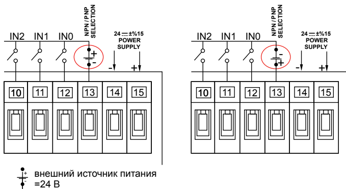
Рисунок Б1.12 — схема подключения дискретных входов PNP/NPN типа
