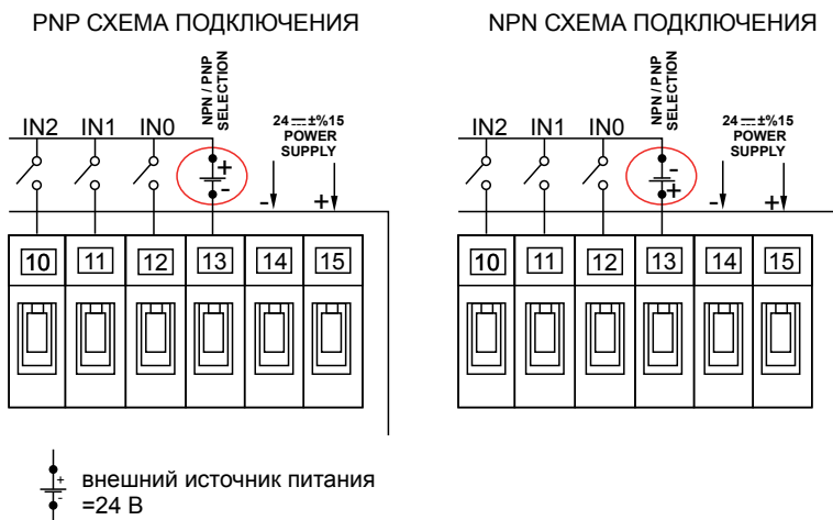
Рисунок Б1.16 — схема подключения дискретных входов PNP/NPN типа
