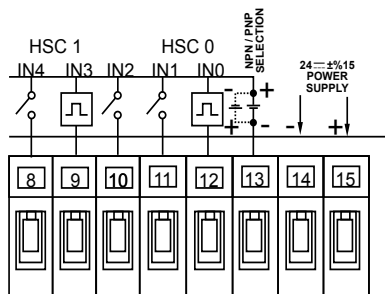
Подключение двух однофазных счетчиков
