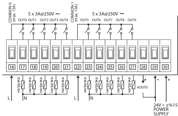
Рисунок Б2.15 - схема подключения нагрузки к релейным выходам
