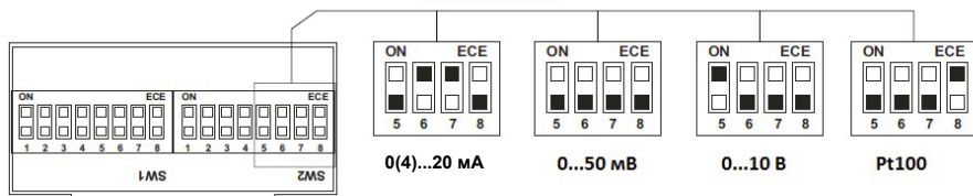
Рисунок Б1.14 - выбор типа входного сигнала DIP переключателями
