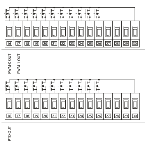
Рисунок Б2.3 - схема расположения PWM/PTO выходов
