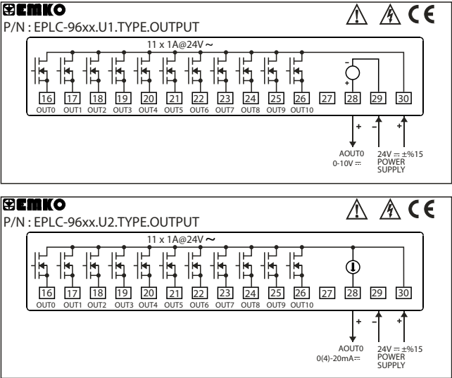
Рисунок Б2.4 - Общая схема подключения модуля вывода «тип U»
