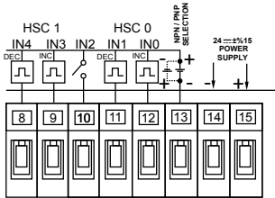
Подключение двух двухфазных счетчиков
