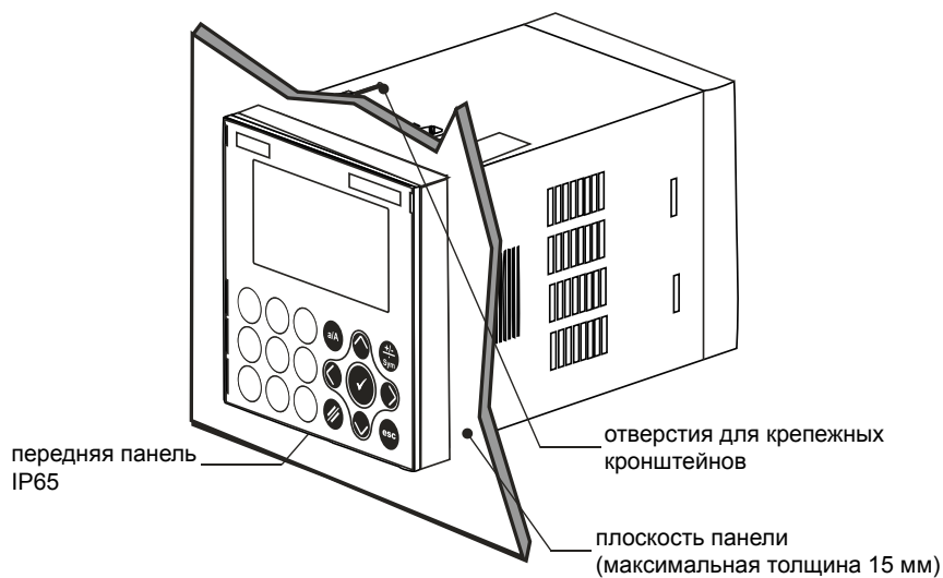
Рисунок 5.1 — внешний вид контроллера EPLC96
