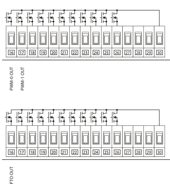
Рисунок Б2.10 - схема расположения PWM/PTO выходов
