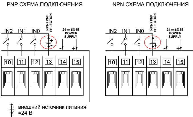
Рисунок Б1.8 — схема подключения дискретных входов PNP/NPN типа
