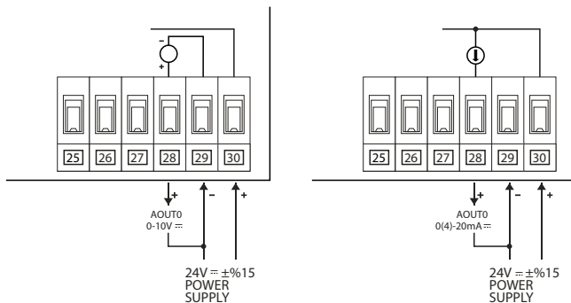
Рисунок Б2.16 - схема подключения нагрузки к аналоговым выходам
