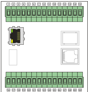
Рисунок 14.5 — расположение порта Ethernet
