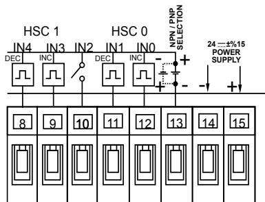
Подключение двух двухфазных счетчиков
