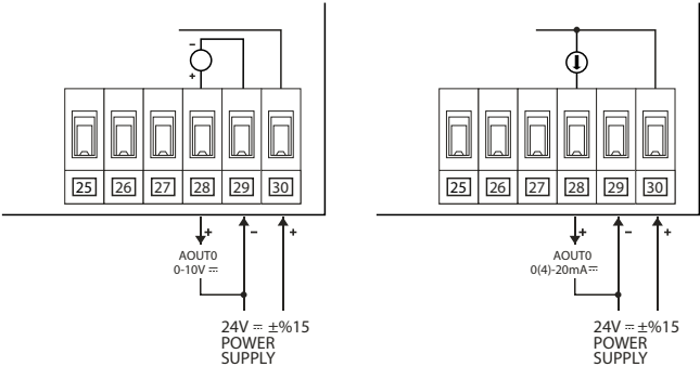
Рисунок Б2.21 - схема подключения нагрузки к аналоговому выходу
