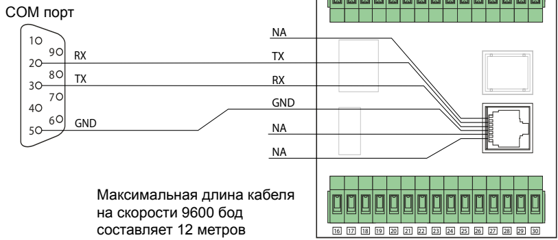
Рисунок 14.1 — раскладка кабеля связи и расположение порта RS-232
