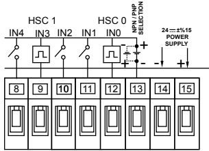
Подключение двух однофазных счетчиков
