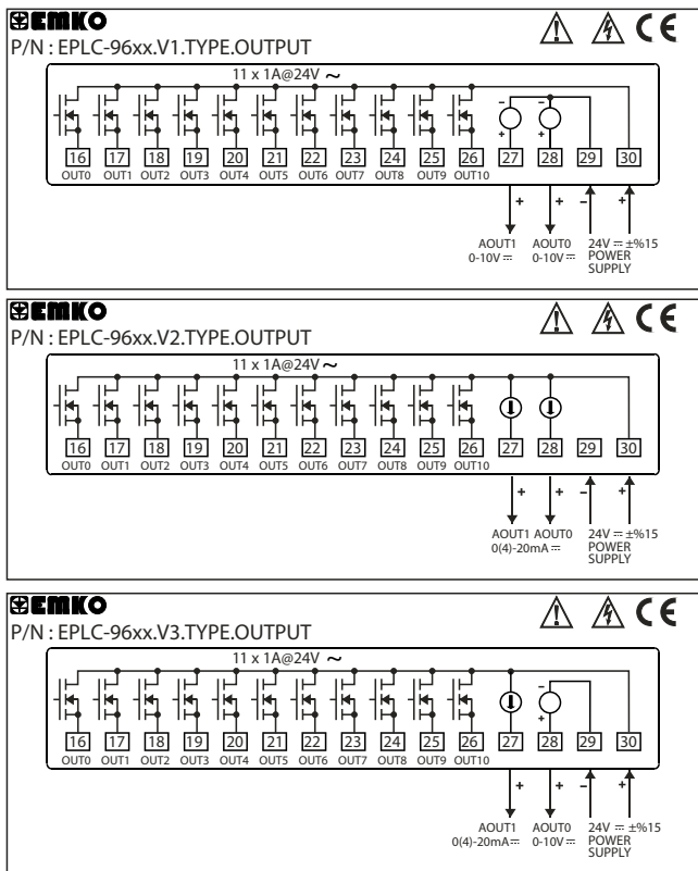
Рисунок Б2.8 - Общая схема подключения модуля вывода «тип V»
