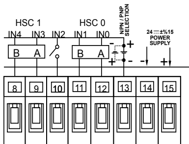
Подключение двух энкодеров (открытый коллектор)
